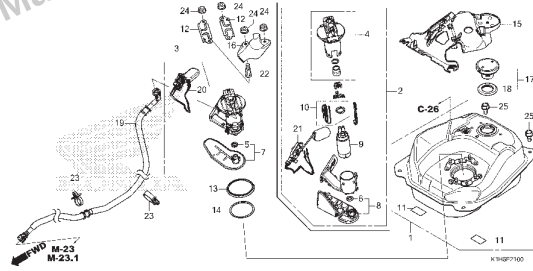
C-21 Tanque de Combustível
