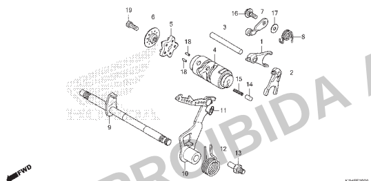
M-19 Tambor Seletor de Marchas
