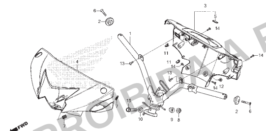
C-7 Guidão • Tampa do Guidão
