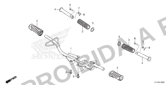
C-30 Pedal de Apoio
