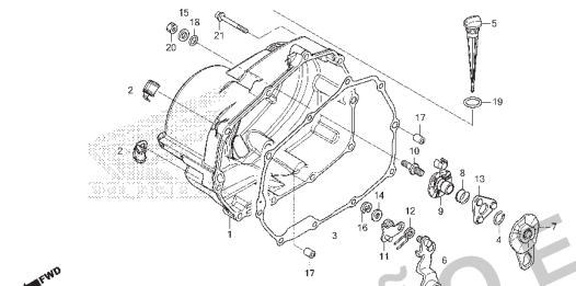
M-9 Embreagem de Partida
