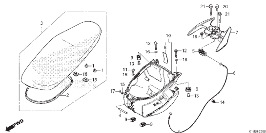
C-26 Câister
