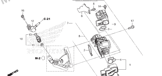
M-23.1 Corpo do Acelerador (BIZ 125 EX)
