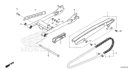
C-32 Garfo Traseiro
