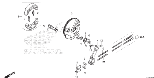
C-18 Painei do Freio Traseiro
